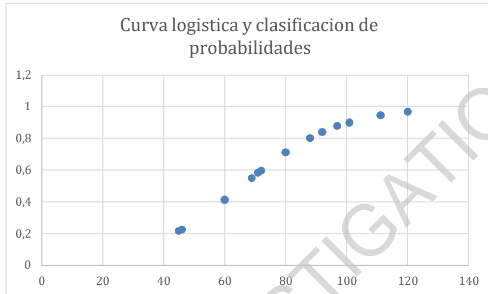
Figura 2. Grafica de la función logística y clasificación de probabilidades de Real Stat
