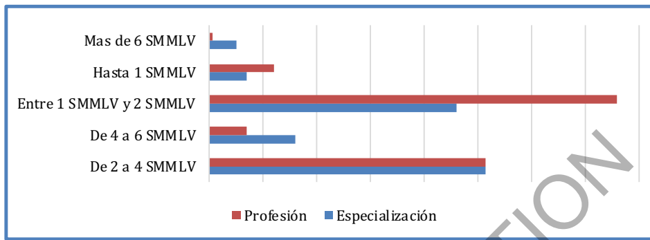
Figura 2. Ingreso Salarial
